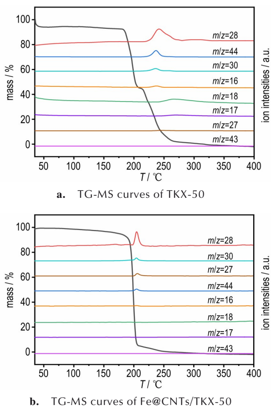
图12 TKX-50和6%Fe@CNTs/TKX-50的TG-MS曲线( \beta=10 °C·min -1 )
