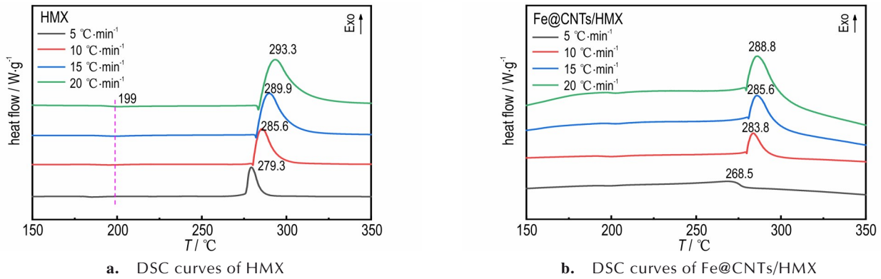
图9 HMX和6%Fe@CNTs/HMX的DSC曲线
