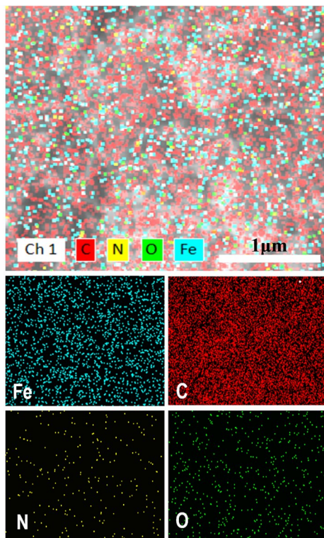
图1 Fe@CNTs的SEM-EDS图
