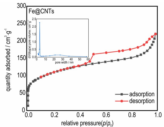
图 6 Fe@CNTs 的 \text{N}_2 吸附-脱附等温曲线和孔径分布图
