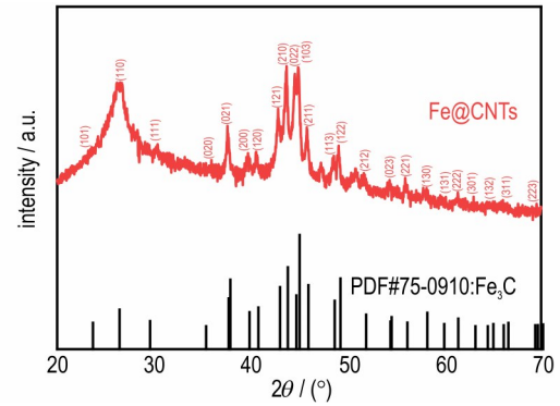
图3 Fe@CNTs的XRD图谱
