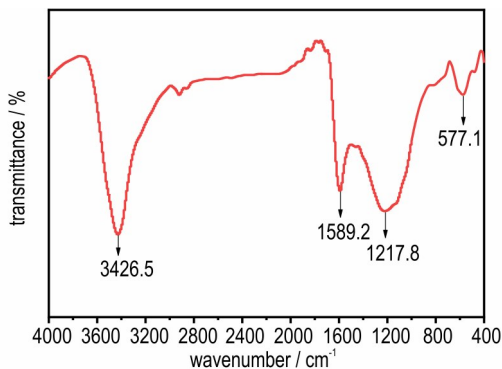
图 5 Fe@CNTs 的红外光谱图
