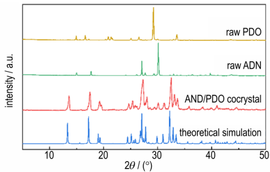
图5 原料及ADN/PDO共晶的PXRD图谱
