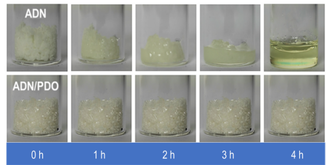
a. hygroscopic changes
