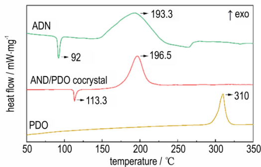
图6 ADN、PDO、ADN/PDO共晶的DSC曲线
