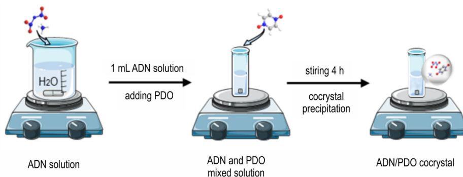
图 2 反应结晶法制备 ADN/PDO 共晶示意图
