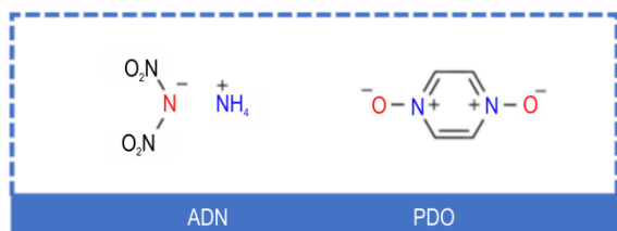
图 1 ADN、PDO 分子结构
