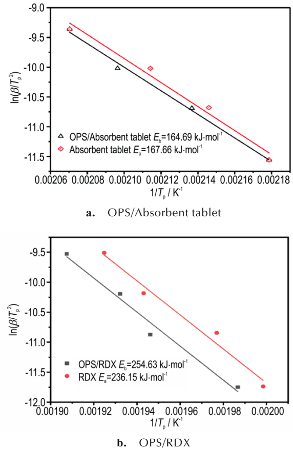
图3 含和不含 OPS 的吸收药片、RDX 的 Kissinger 拟合曲线
