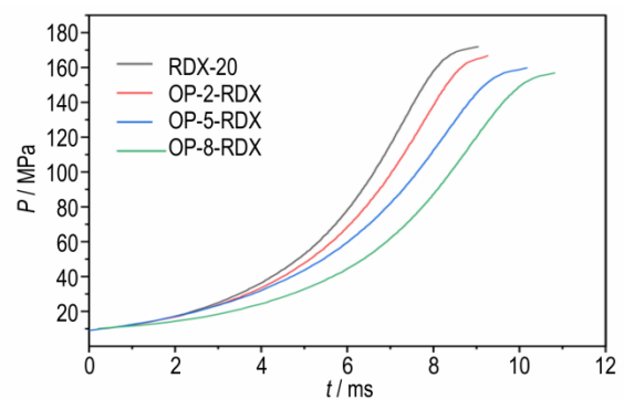
图4 4种不同发射药的 p-t 曲线
