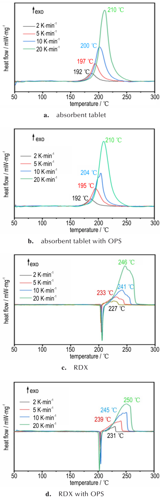
图2 不同升温速率下的DSC曲线
