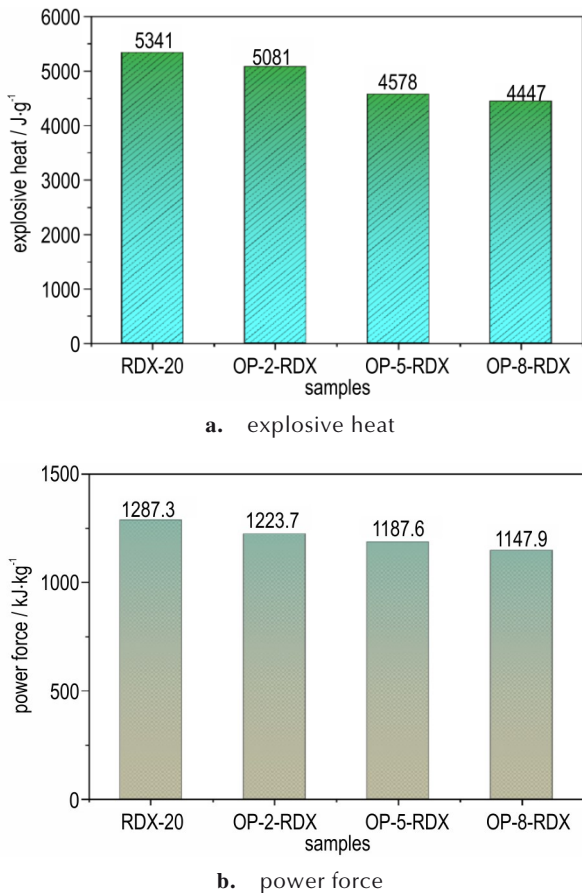
图5 4种不同发射药的爆热和火药力
