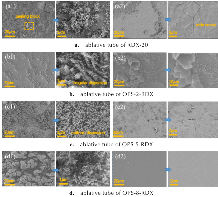
图6 4种不同发射药的烧蚀管内壁表面产物的SEM图
