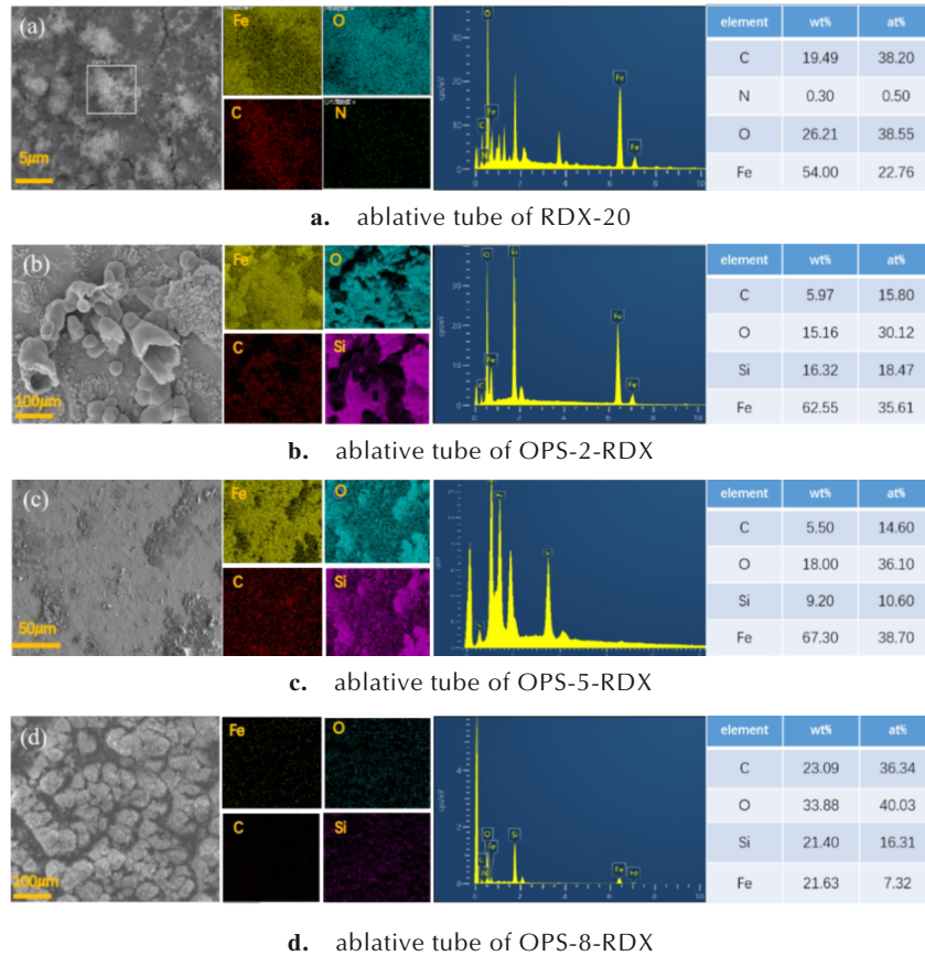
图7 4种不同发射药的烧蚀管内壁表面产物的EDS图像
