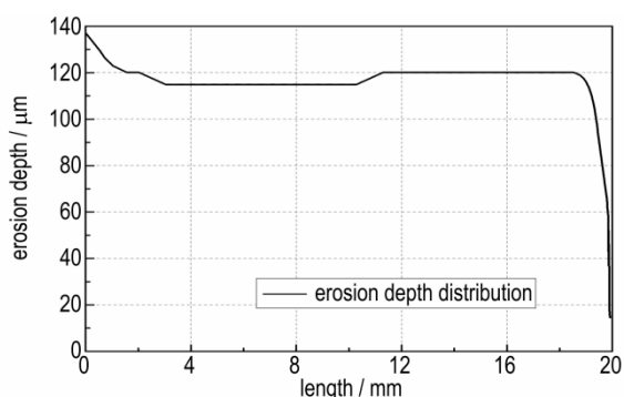
图 6 烧蚀管长度方向烧蚀深度分布
