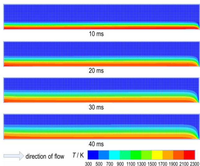
图4 烧蚀管截面温度分布云图
