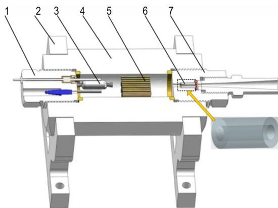
图 1 半密闭爆发器装置图
