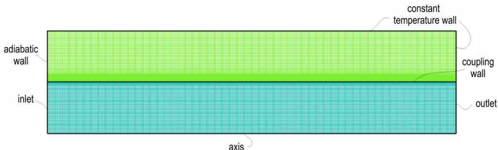
图3 烧蚀管数值计算网格
