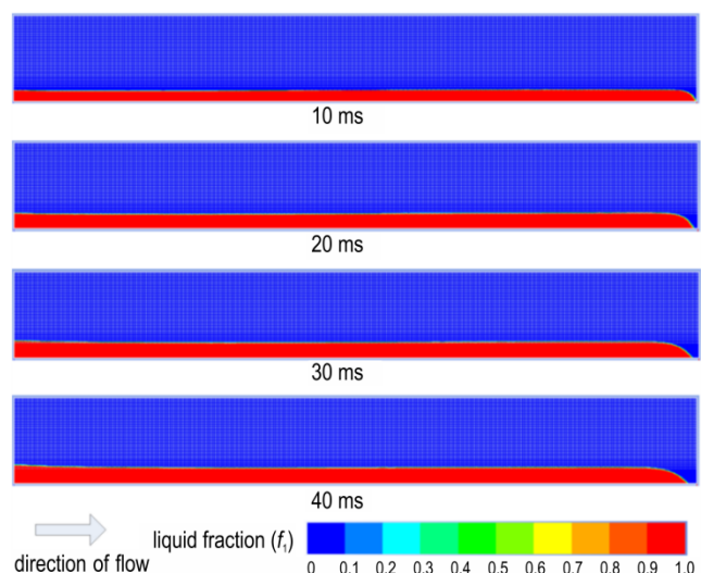
图5 烧蚀管截面液相分数分布云图
