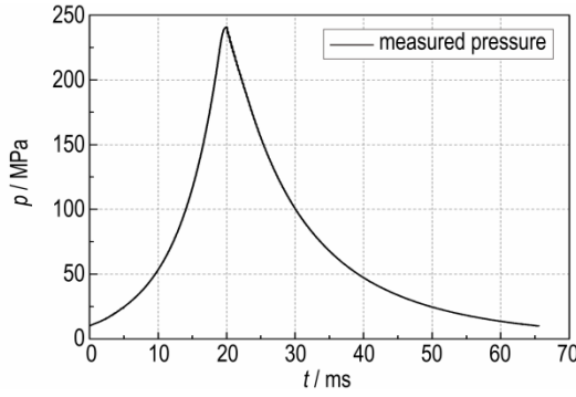
图2 半密闭爆发器试验 p - t 曲线
