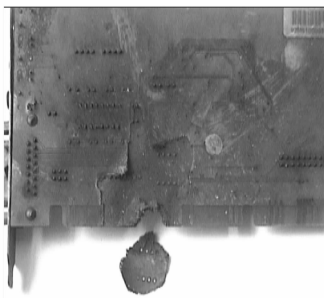
图 7 毁伤增强型破片对铁箱体内电路板的毁伤效果
