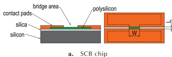
图1 半导体桥芯片结构及封装示意图
