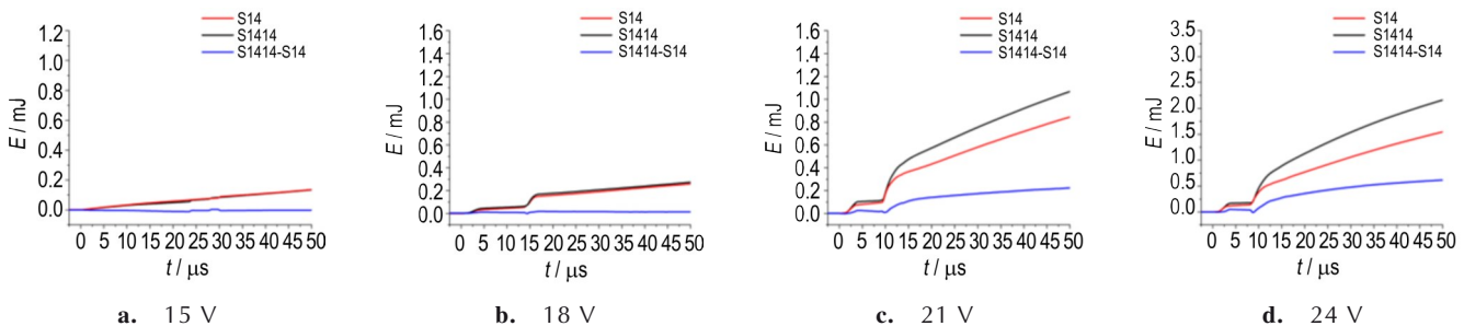
图9 流经AT14型TVS二极管的总能量 E_t 随时间变化图
