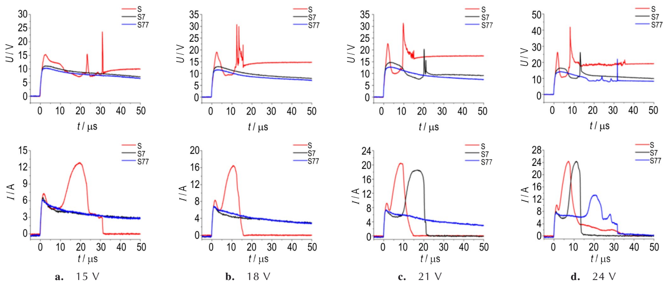
图6 S、S7和S77型样品的电爆曲线
