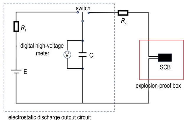
图 5 静电放电电路图 Fig.5 Diagram of electrostatic discharge circuit
