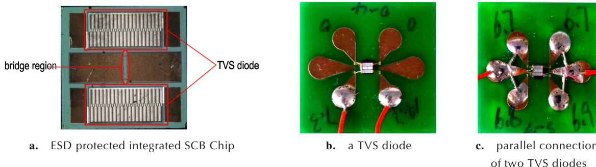
图2 抗静电集成半导体桥芯片及平面TVS二极管结构与连接图
