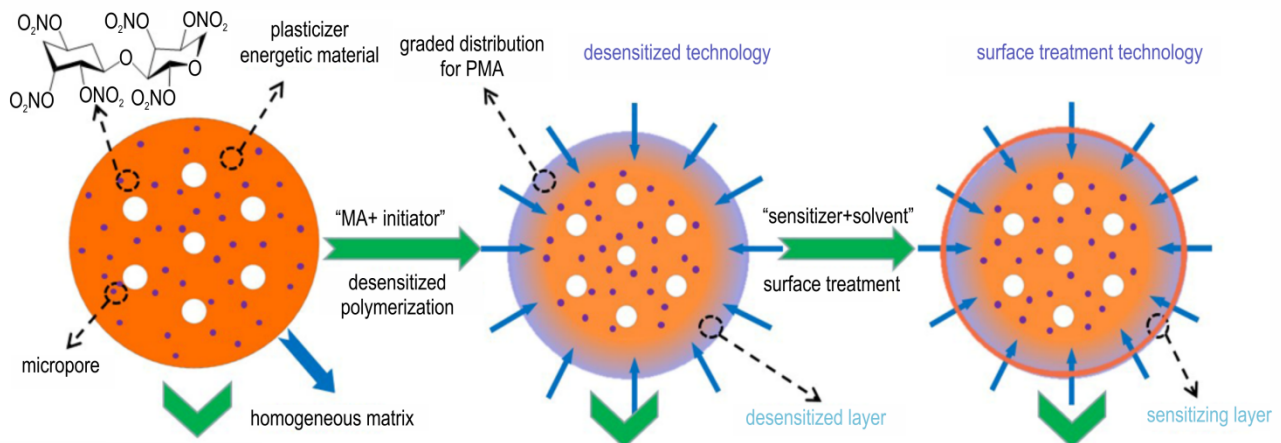
图3 低温度系数调控方案
