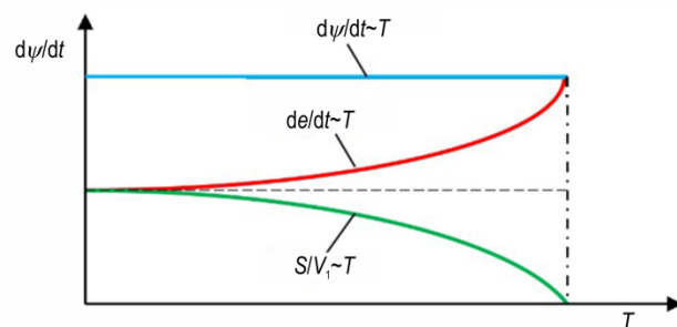
图1 燃面补偿法的调控原理示意图 [10]
