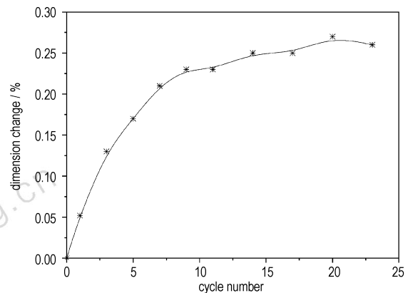
图 1 TATB 基高聚物粘结炸药在热循环过程中的尺寸变化
