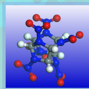
ε-CL-20/PBAMO(9)-g-PAMMO(2)体系的平衡结构
