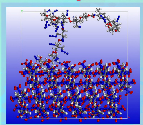
ε-CL-20/PBAMO(9)-g-PAMMO(2)体系的平衡结构
